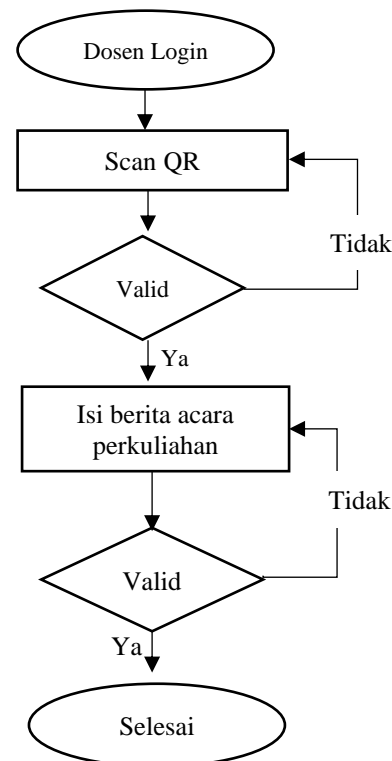
Gambar 19. Flowchart absensi mahasiswa
